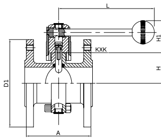
法兰式 (圆形) Flange butterfly valve(Round type)
