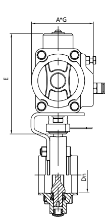
卧式气动蝶阀
