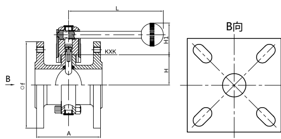
法兰式 (四方法兰) Flange butterfly valve( Square type)
