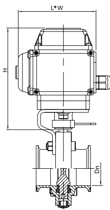
电动蝶阀
